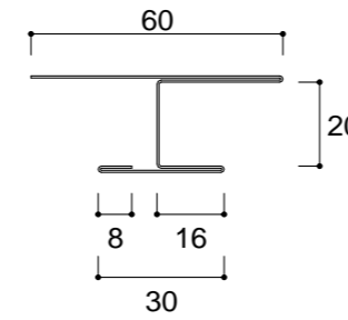
NK - 400 (H型接続) L = 2000 ~ 3000
